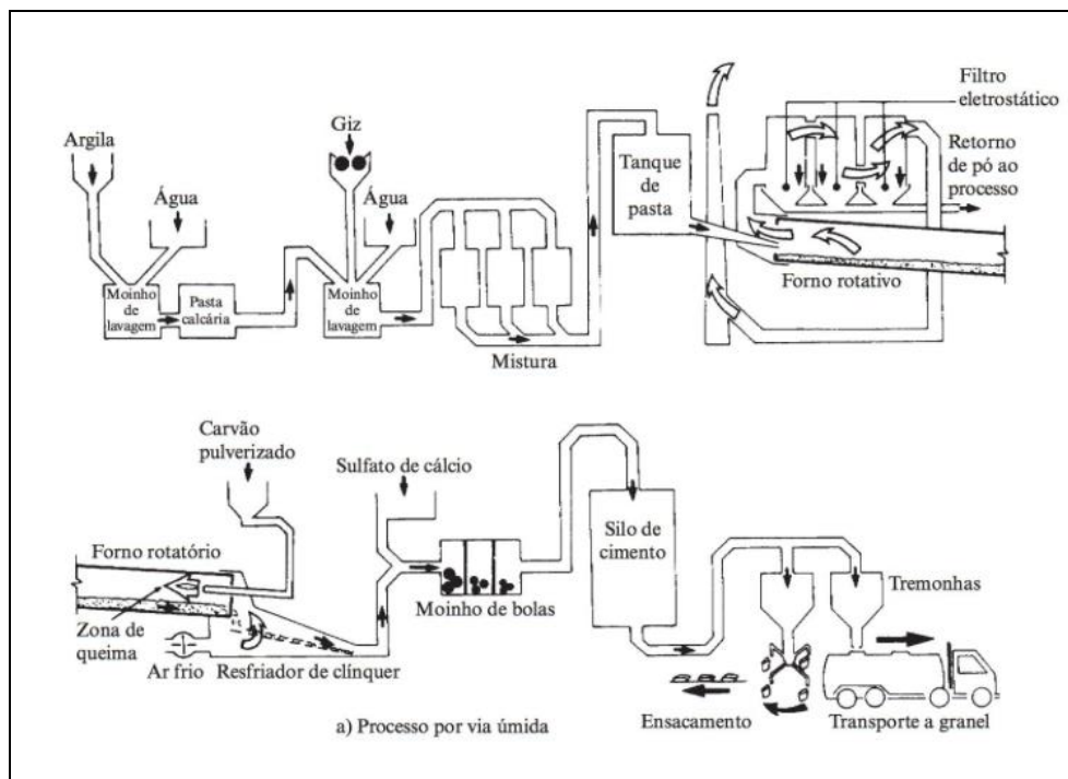
Figura 1- Fluxograma da fabricação do cimento
