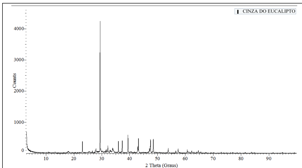
Figura 2: Resultado DRX das Cinzas do Eucalipto
